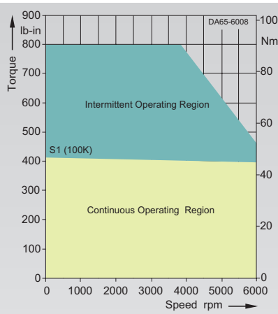
1FT6086-8WK7.-....
