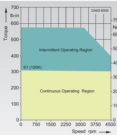
1FT6084-8WH7.-....
