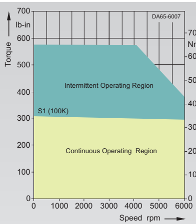
1FT6084-8WK7.-....
