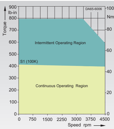
1FT6086-8WH7.-....
